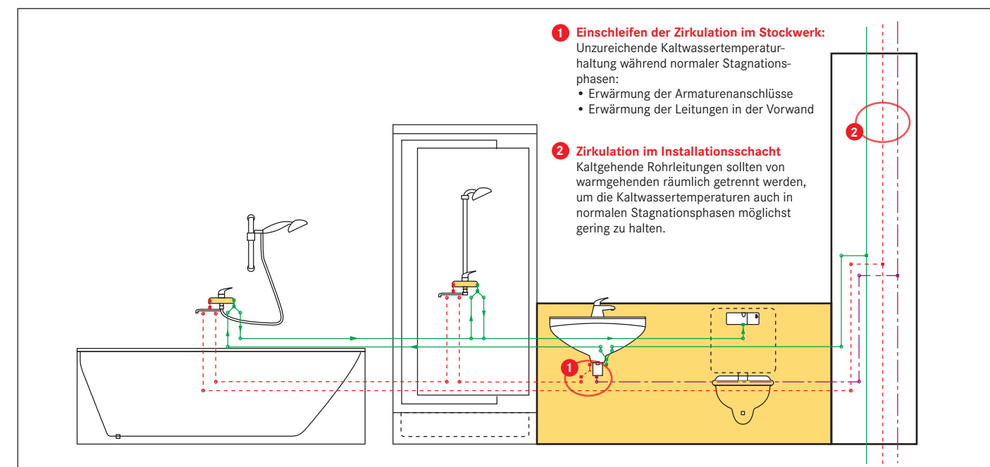
2 – Die Durchschleif-Reiheninstallation mit Warmwasser-Zirkulation erschwert die Temperaturhaltung in der Kaltwasserleitung.
