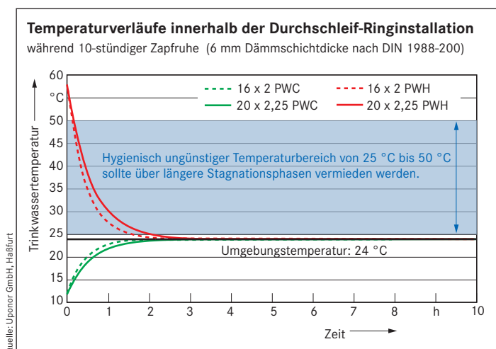
5 – Bei der Durchschleif-Ringinstallation fällt die Warmwassertemperatur aufgrund der fehlenden Zirkulation durch das Stockwerk innerhalb von einer bis eineinhalb Stunden auf die Umgebungstemperatur von 20 bis 24 °C zurück.
