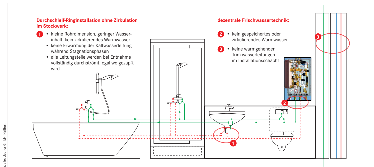
4 – Die Durchschleif-Ringinstallation kommt aufgrund der Parallelschaltung aller Rohrnetzwidestände mit der kleinstmöglichen Rohrdimension und einem nicht zirkulierendem Warmwasserinhalt < 3 l aus.
