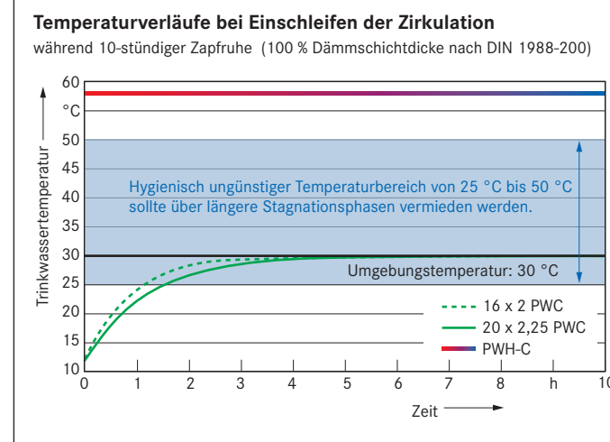
3 – Bei der eingeschleiften Zirkulation erreicht das Kaltwasser trotz normenkonformer 100 %-iger Dämmdicke bereits nach 2 h eine Temperatur von mehr als 25 °C.
