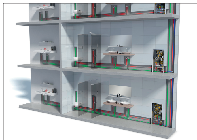
1 – Die Kombination von Wohnungsstationen mit der Durchschleif-Ringinstallation sorgt für die Einhaltung der geforderten Temperaturen sowie einen regelmäßigen Wasseraustausch.
