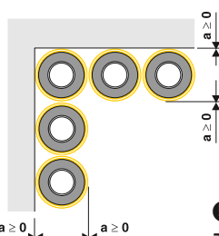
Prinzipskizze für Abstandsregelung bei Wand und Decke
