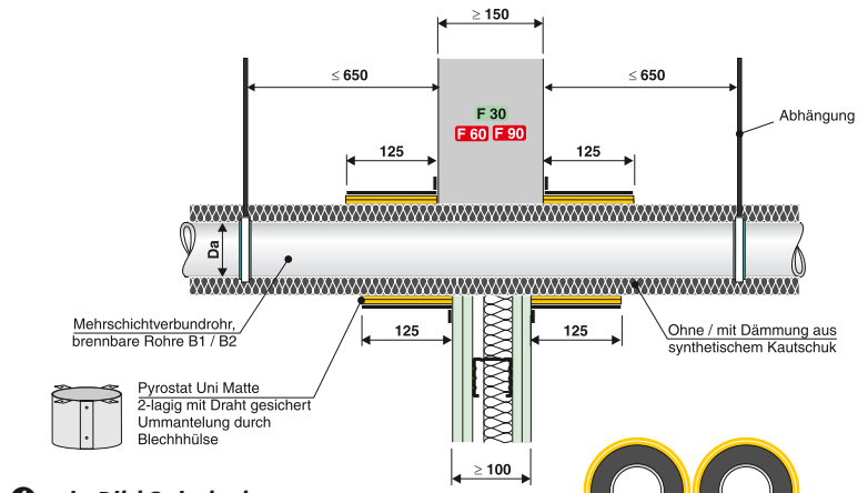
4 wie Bild 3, jedoch nachträgliche Montage
