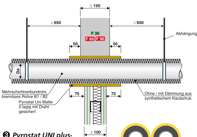
3 Pyrostat UNI plus-K Abschottung bis d \leq 110 mm für brennbare Rohre mit Dämmung aus synthetischem Kautschuk
