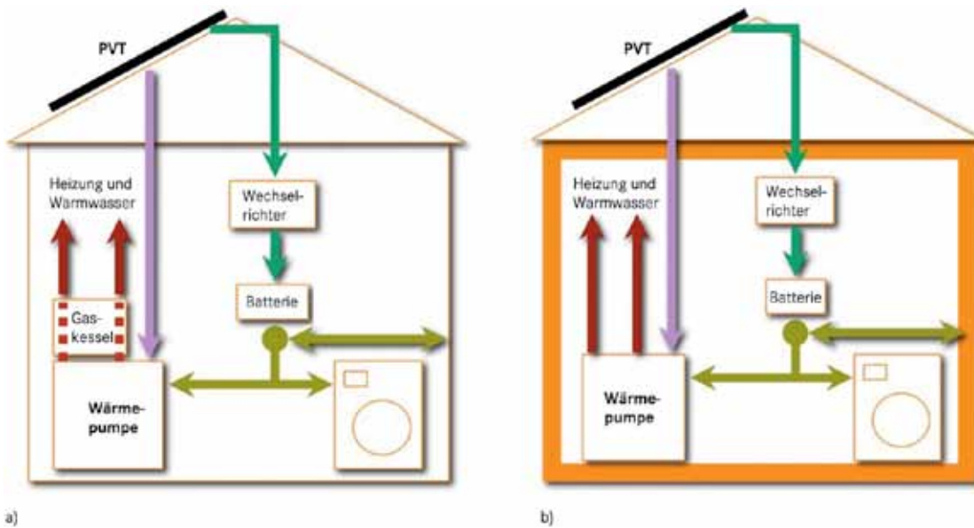
a) Zweistufige Sanierung: links: unsanierte Gebäudehülle mit erster Sanierungsstufe über PVT-Wärmepumpe kombiniert mit Spitzenlast-Gas- bzw. Ölkessel; rechts gedämmtes Gebäude, vollständige Wärmeversorgung mit PVT-Wärmepumpe
