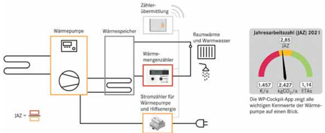
Funktionsschema WP-Cockpit: Die über ein kostengünstiges Zählerset erhobenen Daten werden an die WP-Cockpit-App übermittelt. Die Messergebnisse werden validiert und anonymisiert bereitgestellt, um es allen Interessierten zu ermöglichen, anhand der gewonnenen Daten die Effizienz von Wärmepumpensystemen zu ermitteln, zu bewerten und ggf. zu optimieren.
