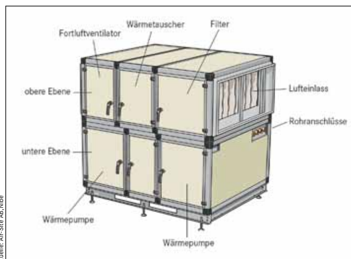
Geräteaufbau des kompakten Nibe/Air-Site Systems
