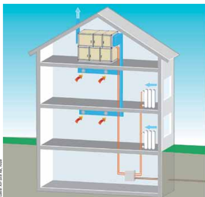
Geräteaufbau des kompakten Nibe/Air-Site Systems
